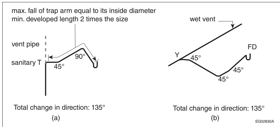
Figure A-2.5.6.3.(1)-B
