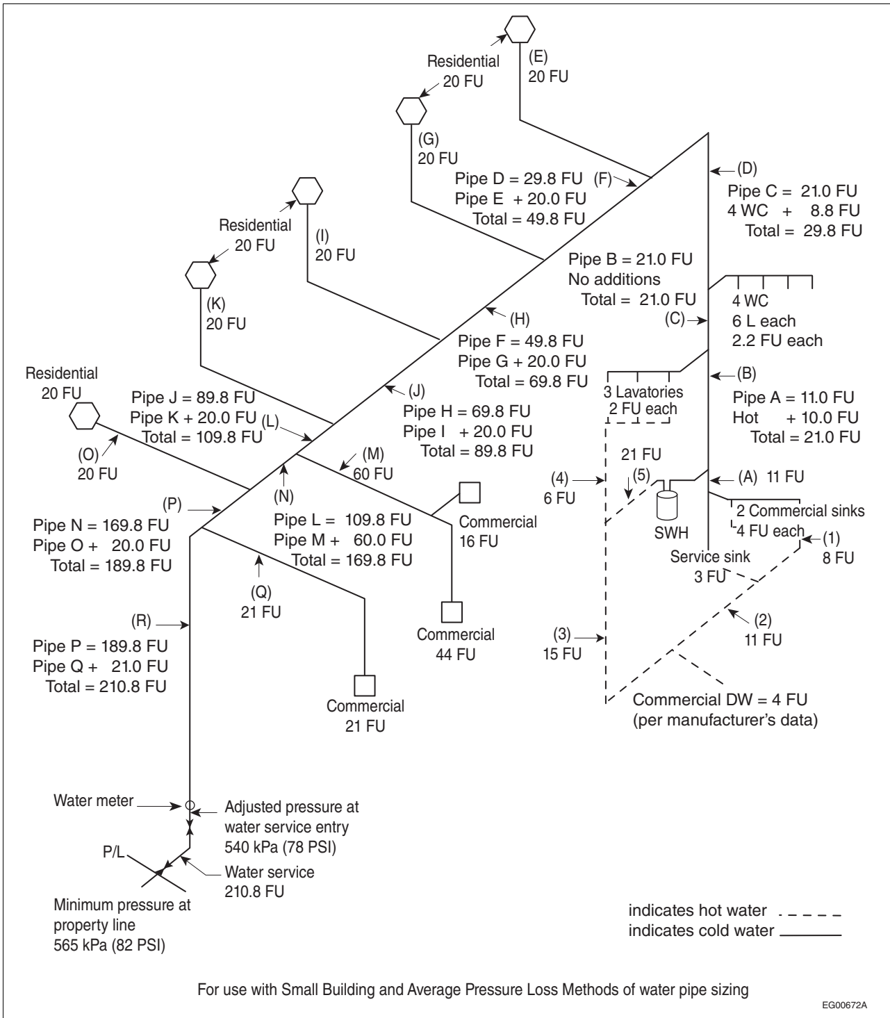
Figure A-2.6.3.1.(2)-A
